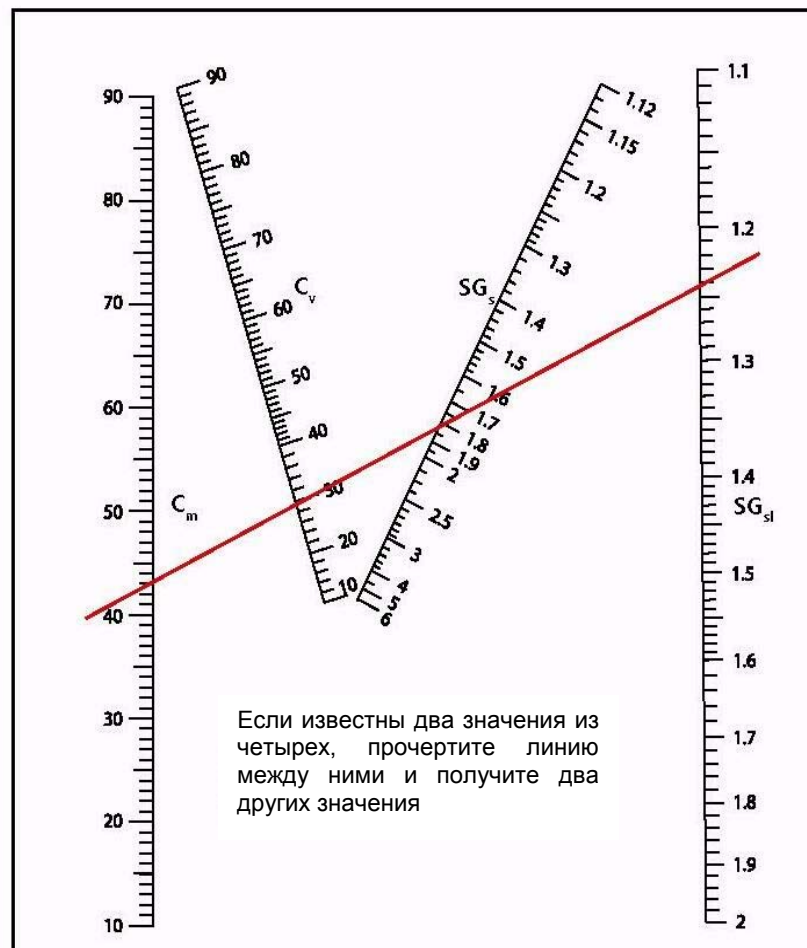
Номография, показывает соотношение концентрации и удельной массы шлама в воде.
